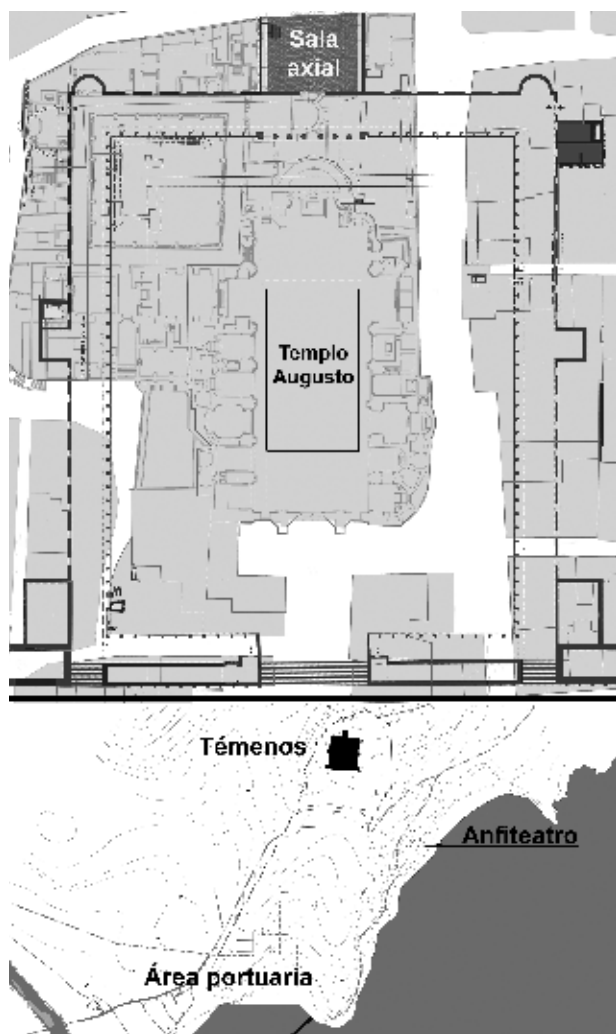
FIGURA 8. Planta del antiguo recinto de culto en su contexto urbano (a partir de Macías et al. 2007).
