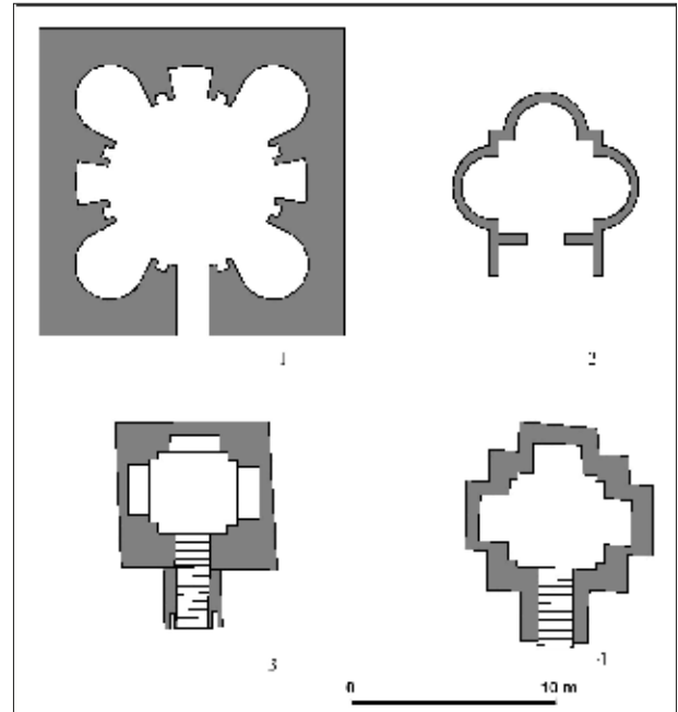
FIGURA 5. Plantes comparatives dels mausoleus. 1. Mausoleu de planta central de la necròpolis; 2. Mausoleu del carrer Sant Auguri; 3. Cripta dels Enginyers; 4. Mausoleu veí a la Cripta dels Enginyers.
