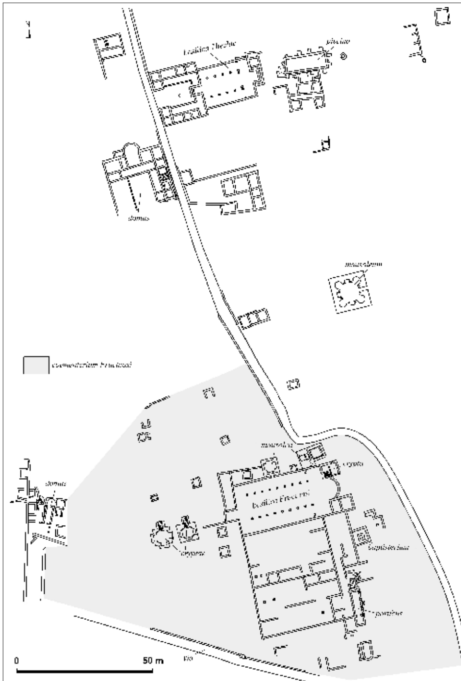
FIGURA 2. Planta general del conjunt paleocristià del Francoquí. Al sud, la basílica martirial de Sant Fructuós amb l'edifici annexat que conté un baptisteri i un pòrtic encarat a la ciutat. Més a l'oest, dues criptes i les restes d'una domus tardoromana. Seguint la via cap al nord hi ha, a la dreta, les restes d'un gran mausoleu de planta central. Més amunt apareix representat el conjunt descobert l'any 1994: a l'esquerra, la domus del segle IV; a la dreta, un grup d'edificis del segle V entre els quals ressaltava la basílica de Thecla amb el seu atri (López 2006).
