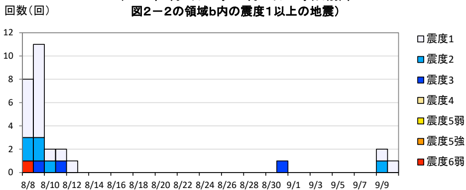
図1-1 震度1以上の日別地震回数グラフ
